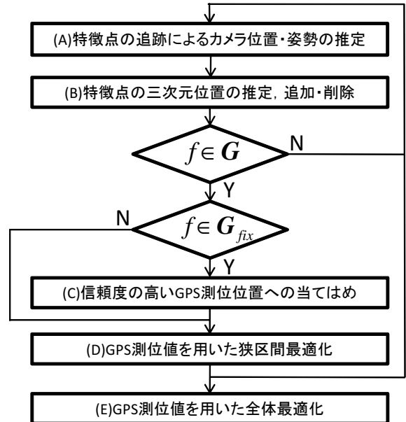
図2 提案手法の処理の流れ
