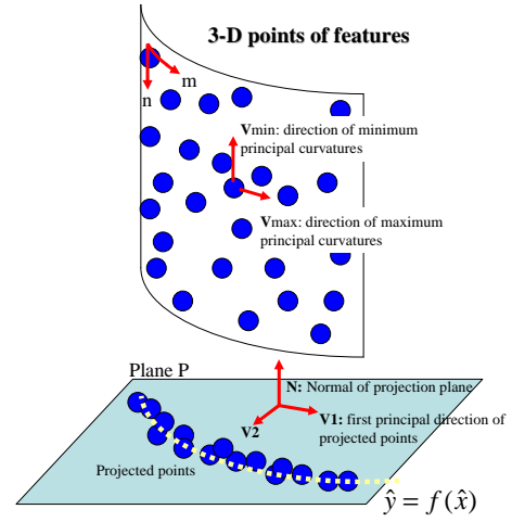
図 4 多項式あてはめによる紙面形状の推定
