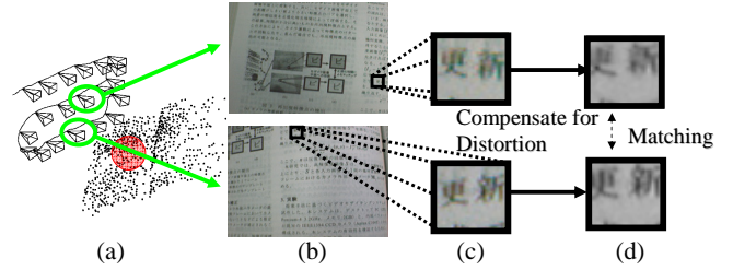
図 3 再出現特徴点の検出; (a) カメラの移動経路と特徴点の三次元位置, (b) 入力画像中の時間的に離れたフレーム, (c) 各画像上における同一特徴点のパターン, (d) 投影歪みの影響を取り除いたパターン
