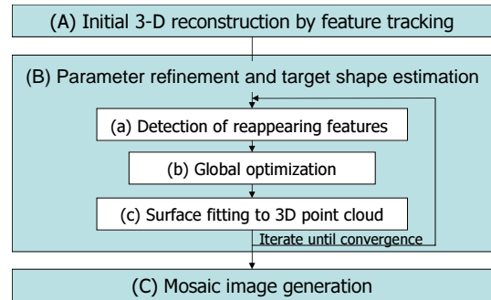
図 2 提案手法の処理の流れ
